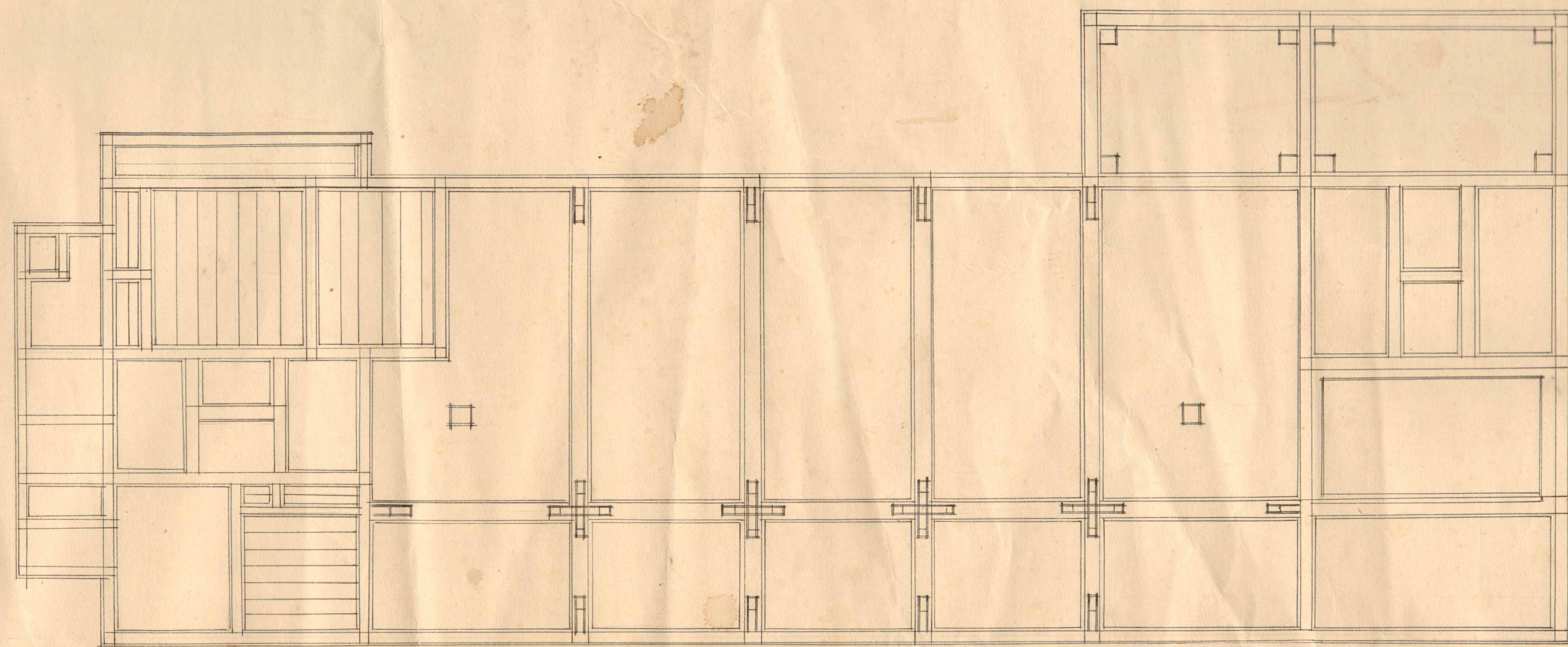
階下天井伏図
