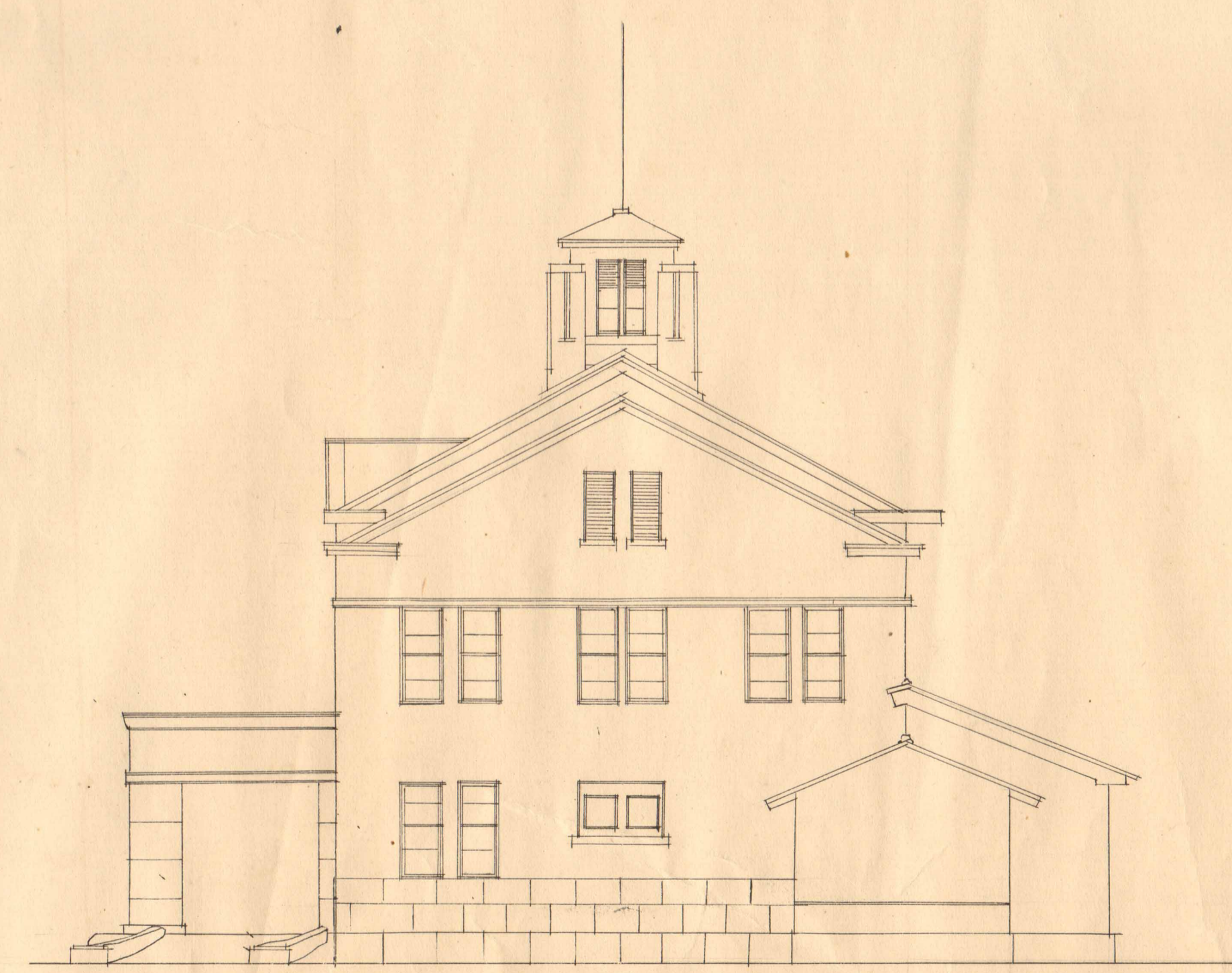
右側面圖
